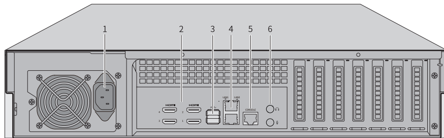
图1-3 TL-TUMS2500后面板示意图
