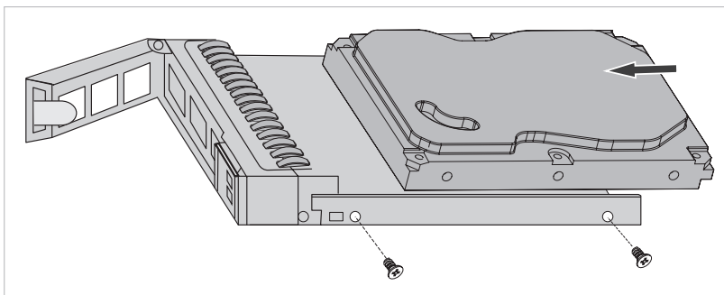
图3-2 安装硬盘
