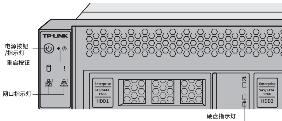
图1-2 前面板按钮与指示灯
